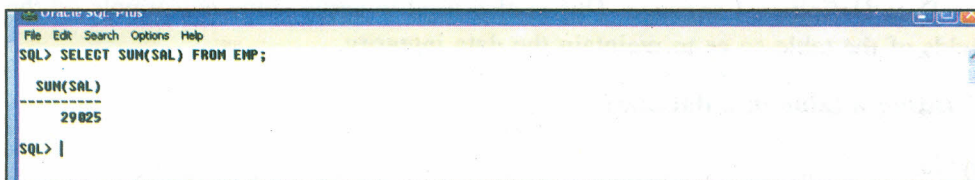
Fig. 30: Sum function
